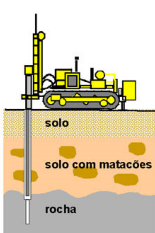
Equipamento de perfuração de estacas raiz
