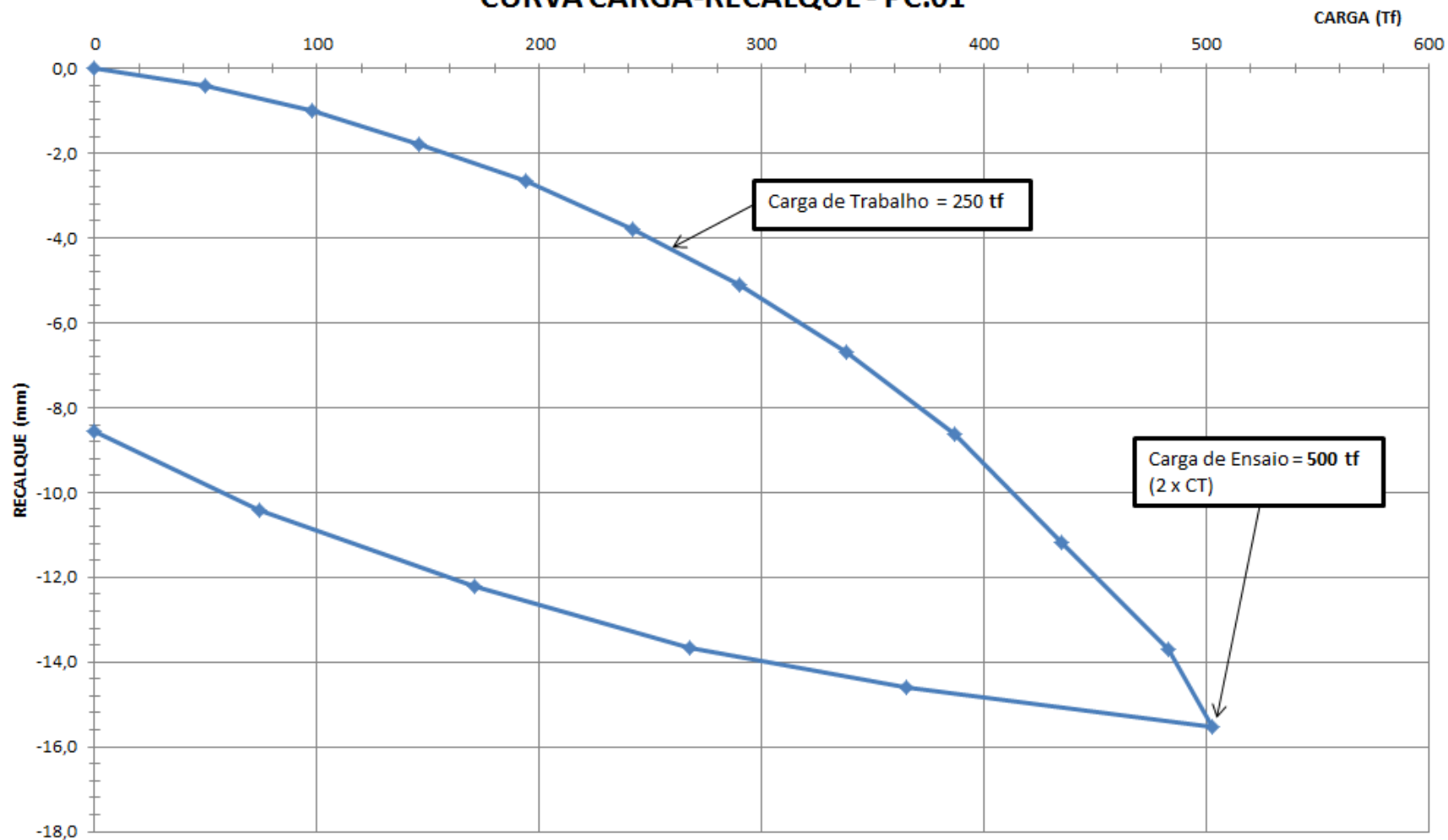
CURVA CARGA-RECALQUE - PC.01
