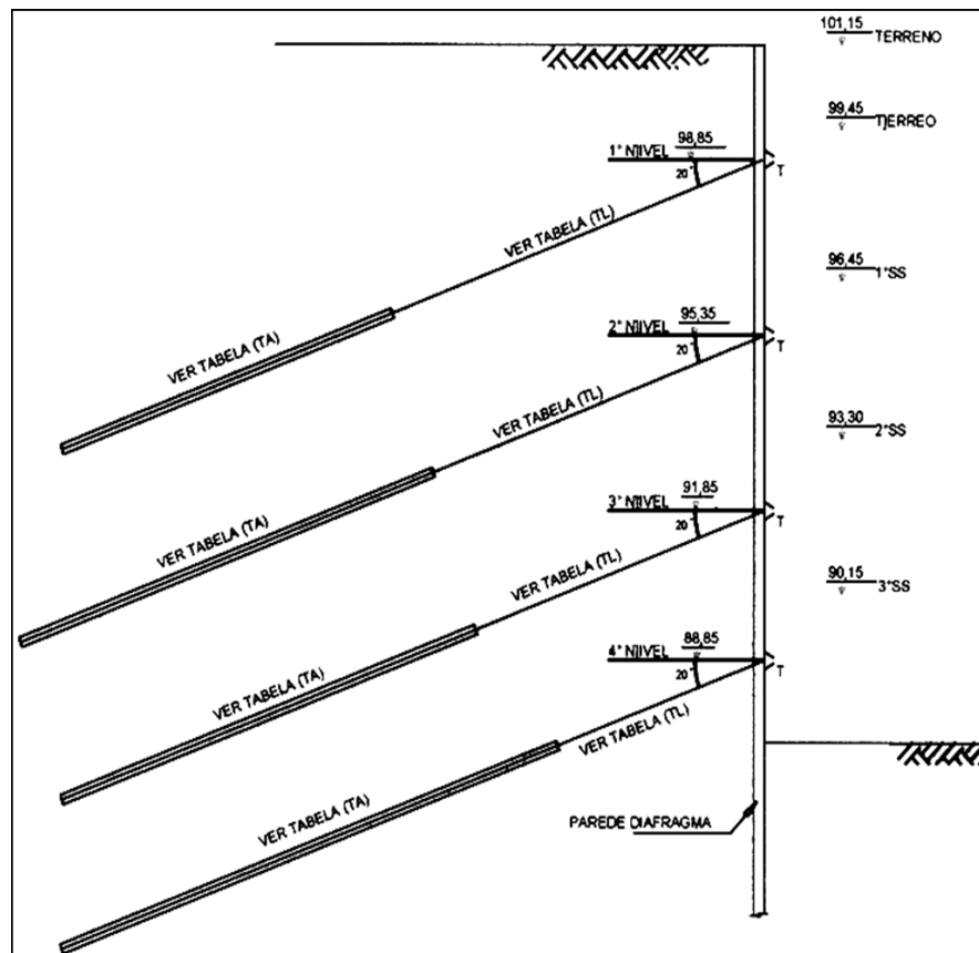
Corte esquemático dos tirantes provisórios
