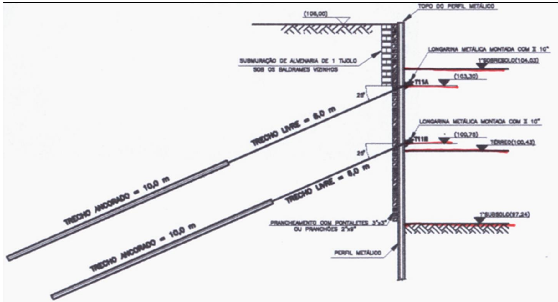
Corte B-B
