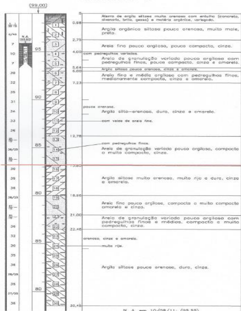
SONDAGEM SP-8
