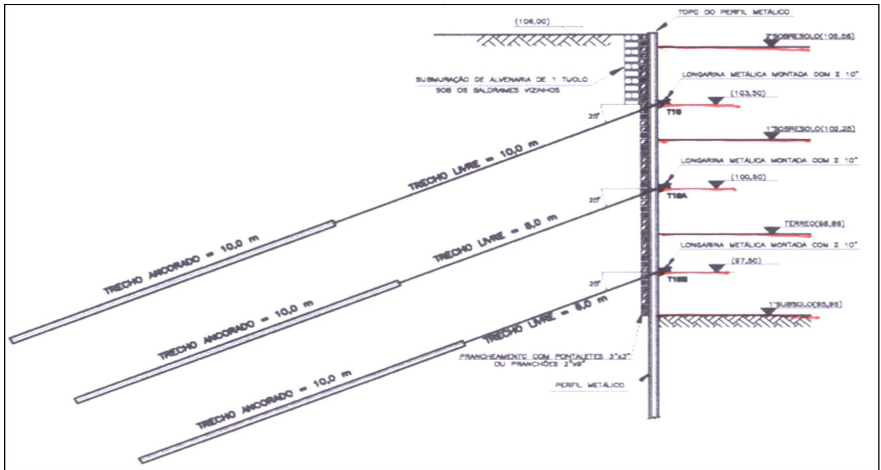
Corte C-C
