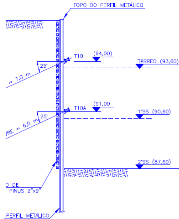
CORTE A-A
