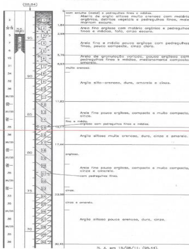
SONDAGEM SP-7
