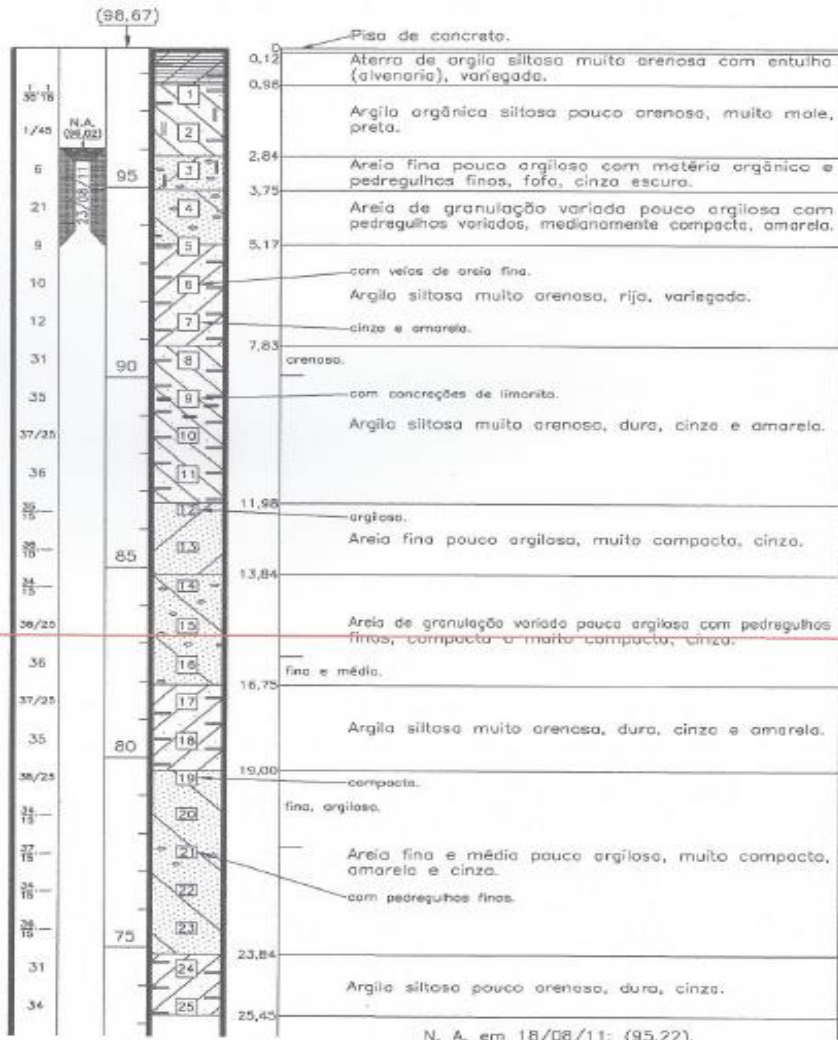
SONDAGEM SP-6
